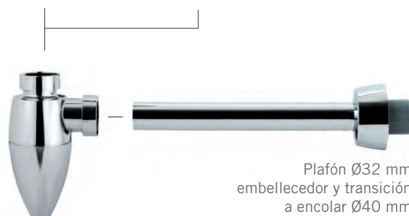
Sifón botella con cuerpo en forma de ánfora en ABS cromo. 1 1/4".
