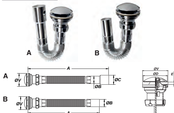
Válvula desagüe con embellecedor Click-Click y tubo flexible cromado.
