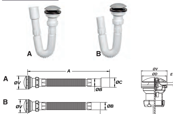
Válvula desagüe con embellecedor Click-Click y tubo flexible blanco.
