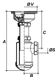
Sifón botella extensible con válvula de cesta.
