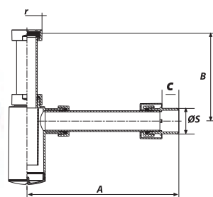
Sifón botella, extensible con alargadera y plafón.
