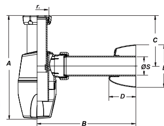
Sifón botella Juntafix, extensible, alargadera y plafón.
