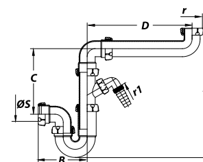
Sifón curvo desplazado con toma electrodoméstico.
