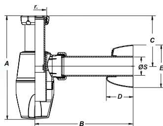
Sifón botella, extensible, salida horizontal, alargadera y plafón.
