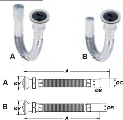
Válvula de Ø70 con tubo flexible cromado.
