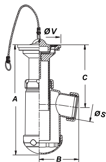
Sifón botella extensible con válvula lavabo-bidé.
