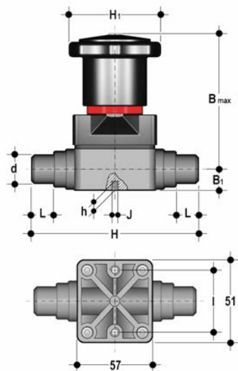
CMDM Válvula de membrana compacta con conexiones macho para soldadura socket, serie métrica
